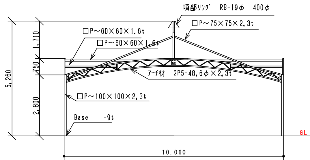
側面図
